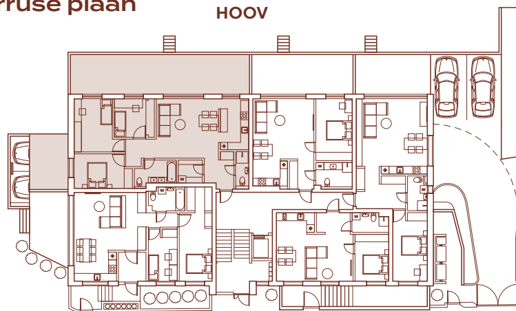
Korruse plaan
